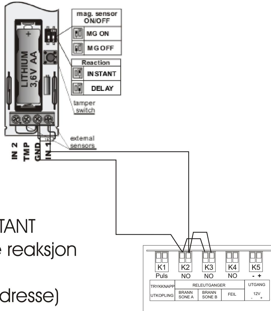
Aspirasjonsdetektor, IRS-3
